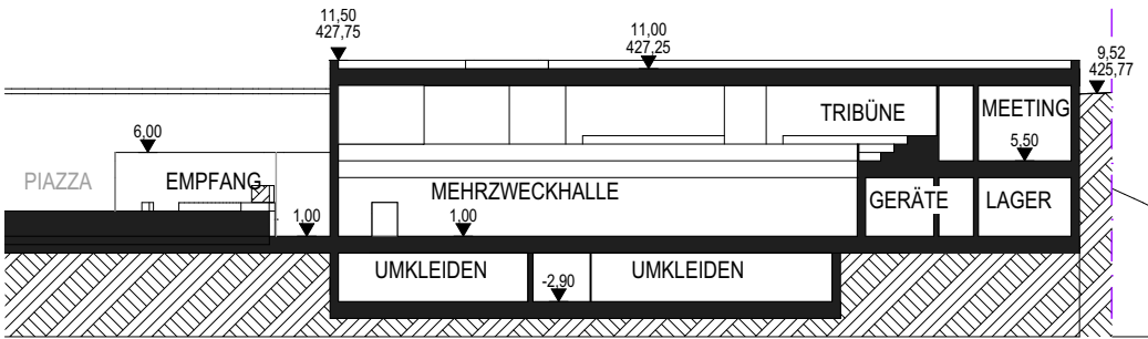
Schnitt Mehrzweckhalle
