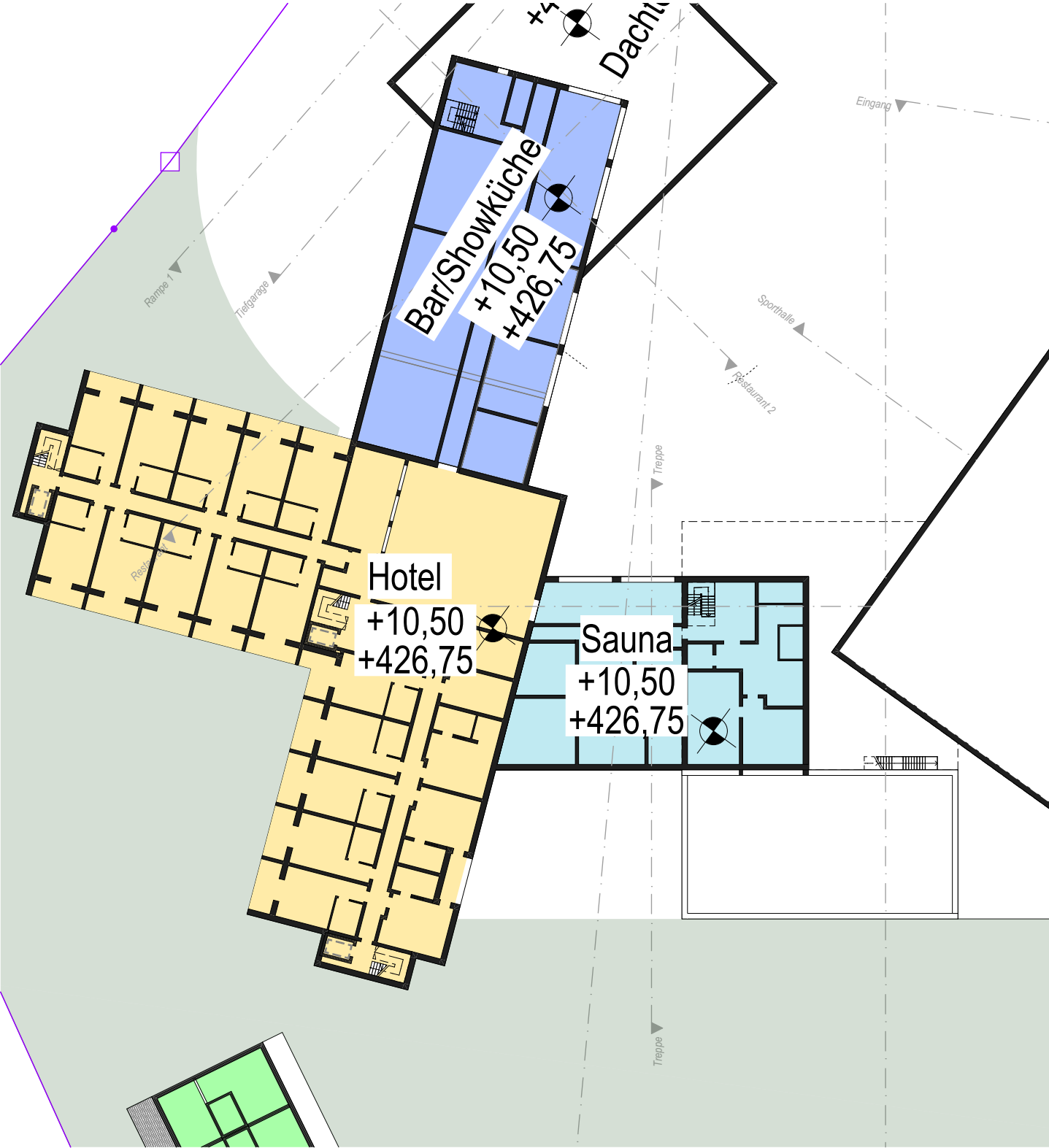
Hotel Obergeschoss 2
