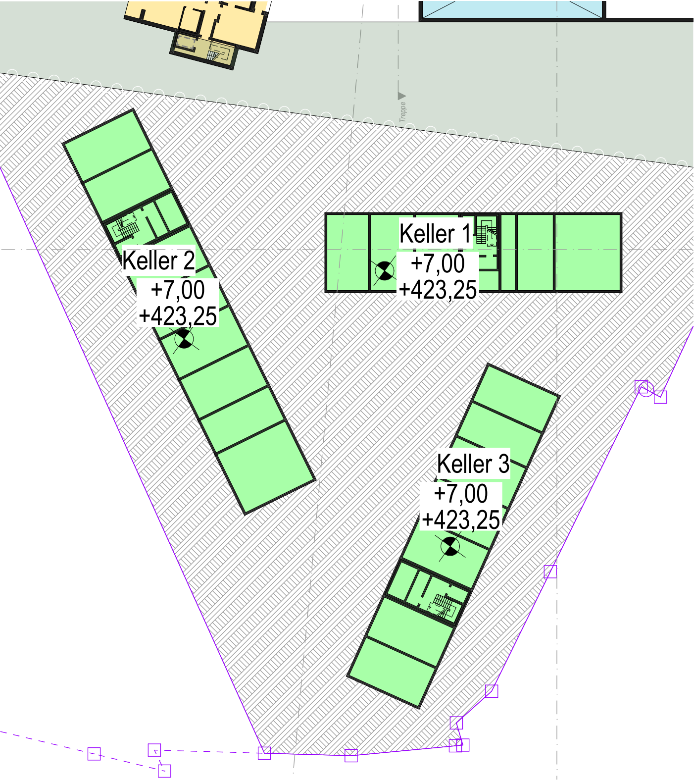
Servicewohnen Keller
