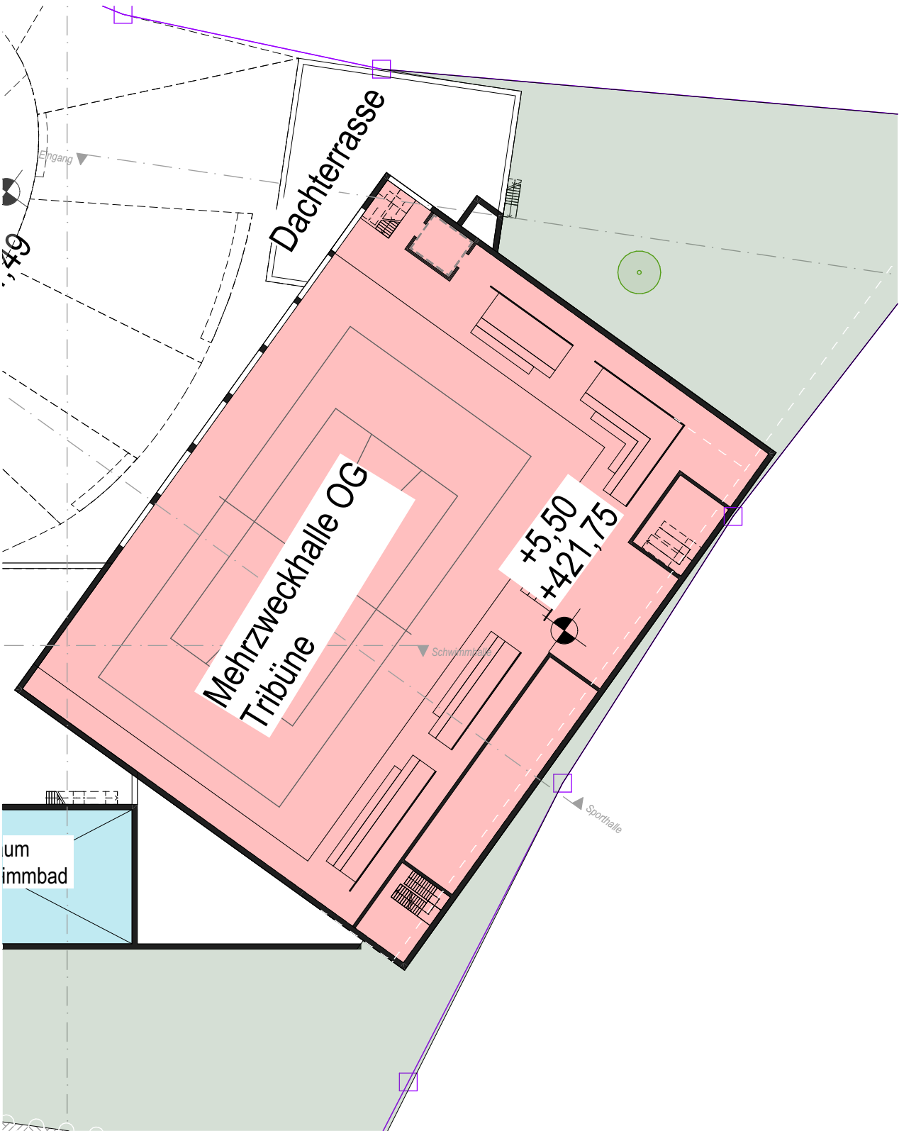
Sportbereich Oberschoss
